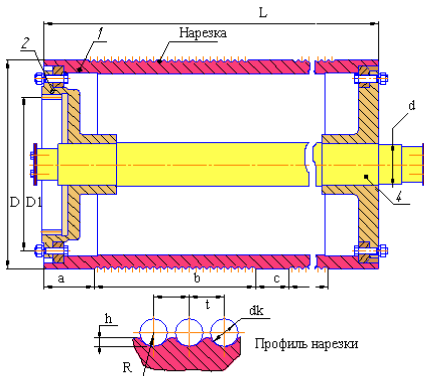
Барабан грузовой крановый: основные размеры
